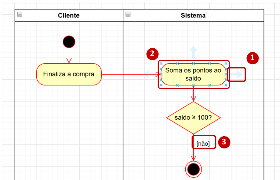
Figura 9 — Ligando as formas: setas azuis (1), pontos de conexão (2) e a guarda escrita na seta (3).
