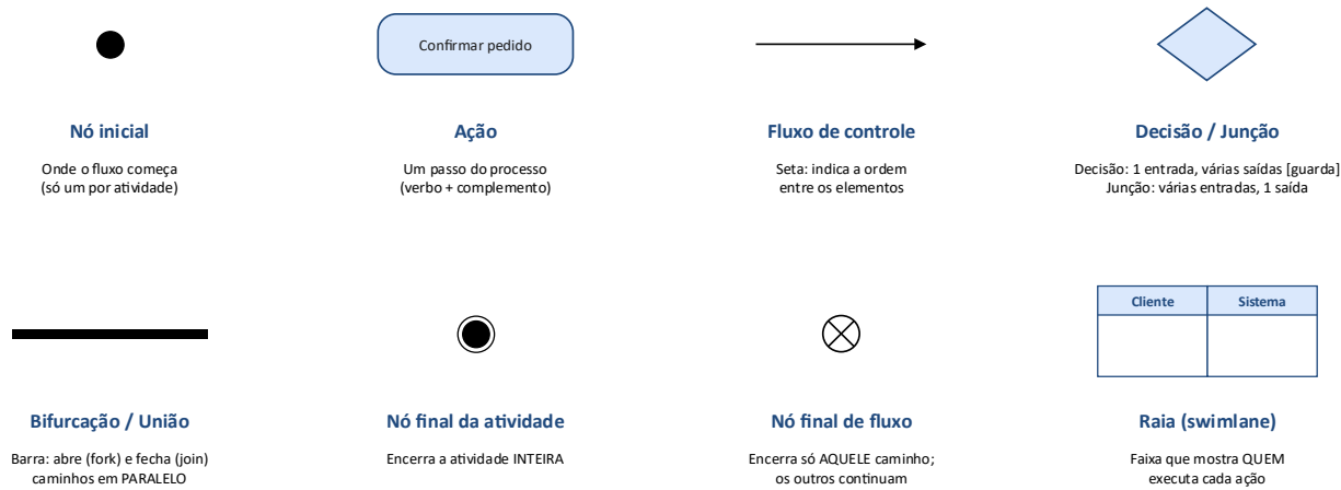
Figura 1 — Os elementos do diagrama de atividades.
