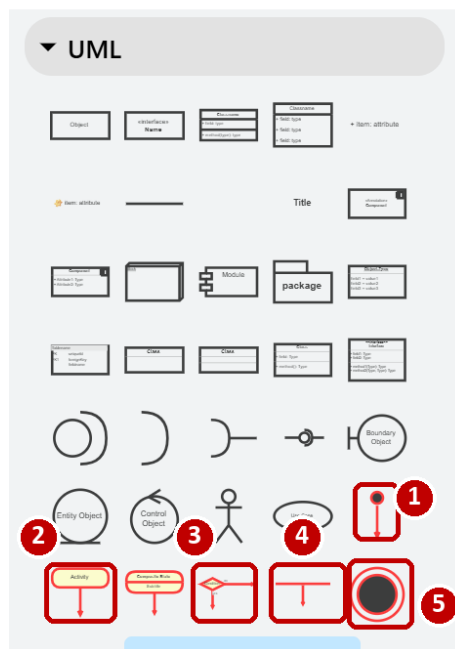
Figura 7 — As formas do diagrama de atividades na paleta UML.
