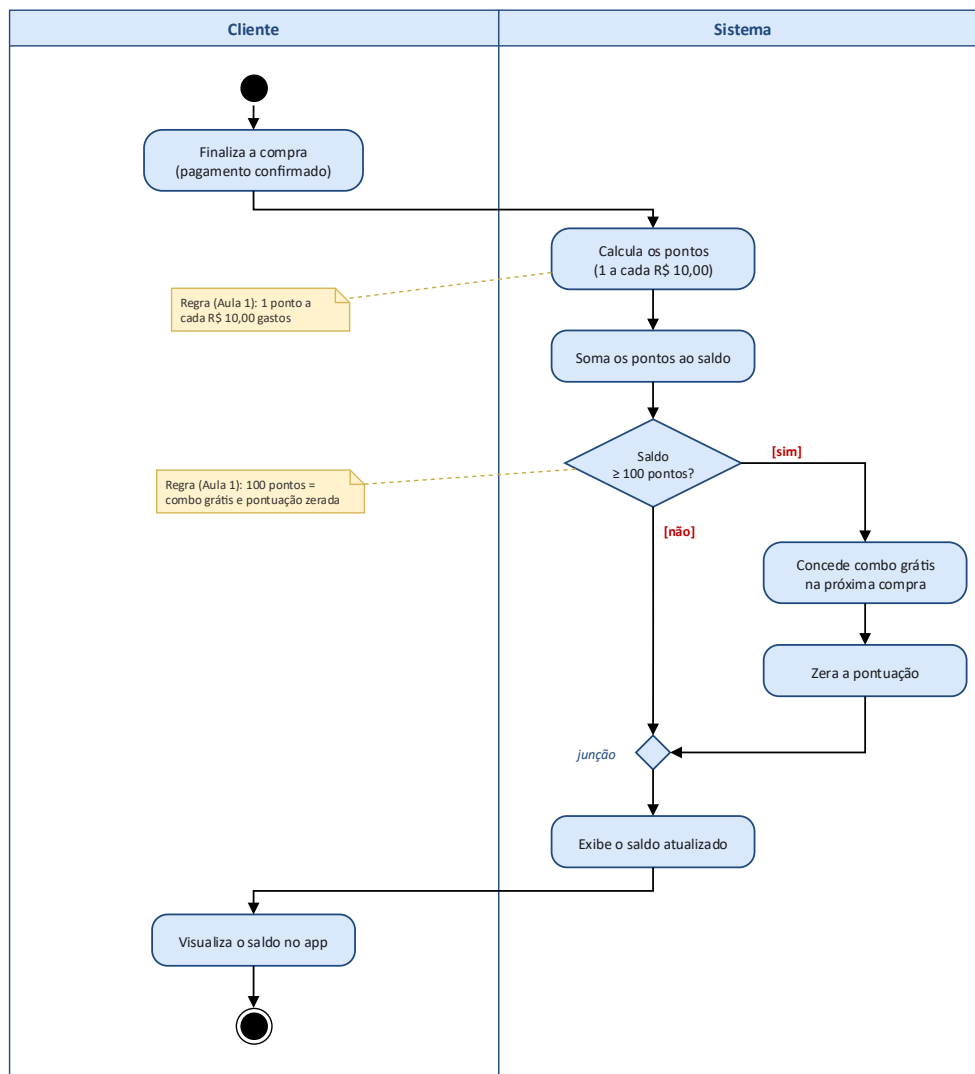
Figura 10 — Resultado do exemplo guiado: acumular pontos de fidelidade.
