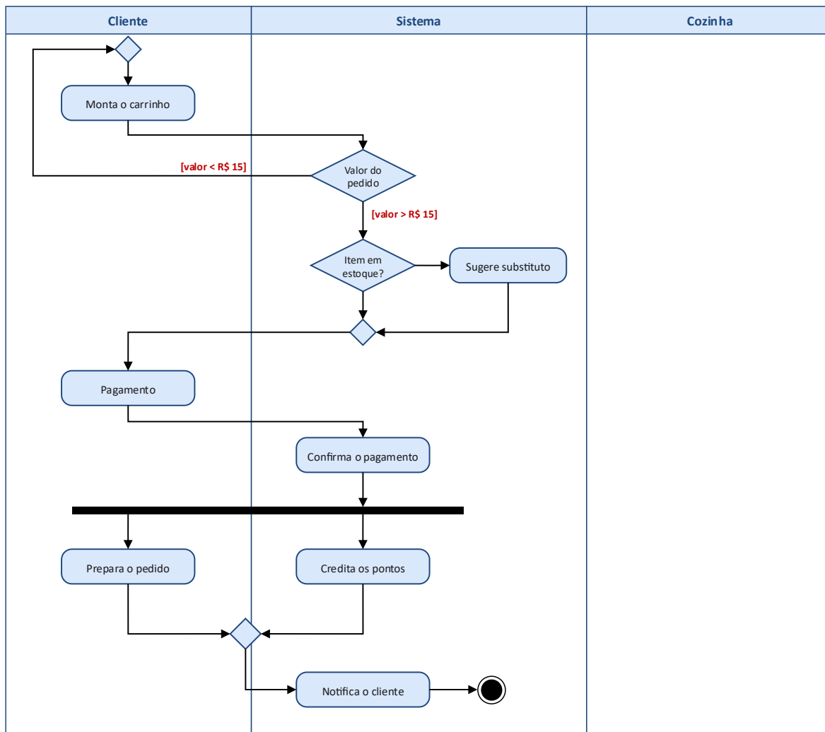
Figura 11 — Diagrama com 6 erros propositalmente.
