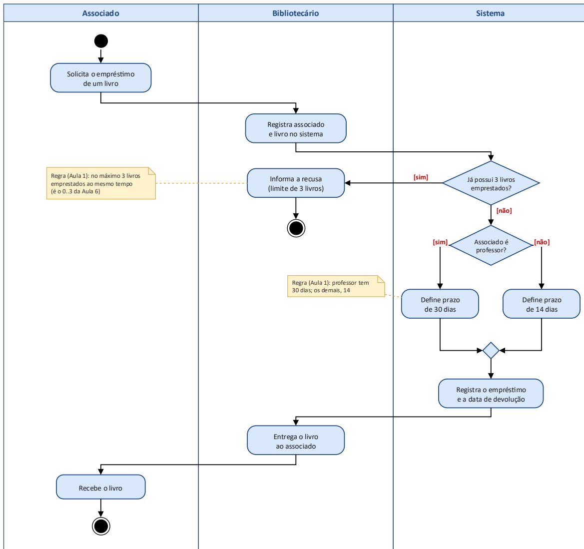
Figura 5 — Biblioteca “Ler Mais”: emprestar um livro.
