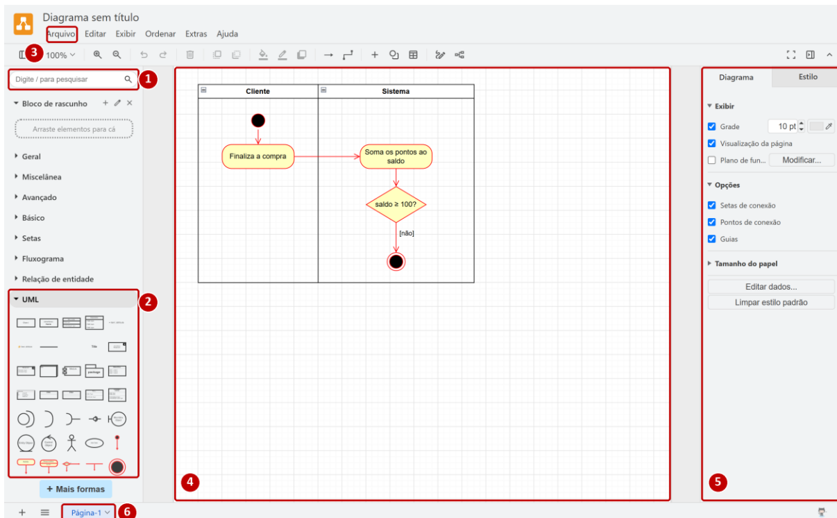
Figura 6 — A tela do draw.io e seus seis lugares principais.
