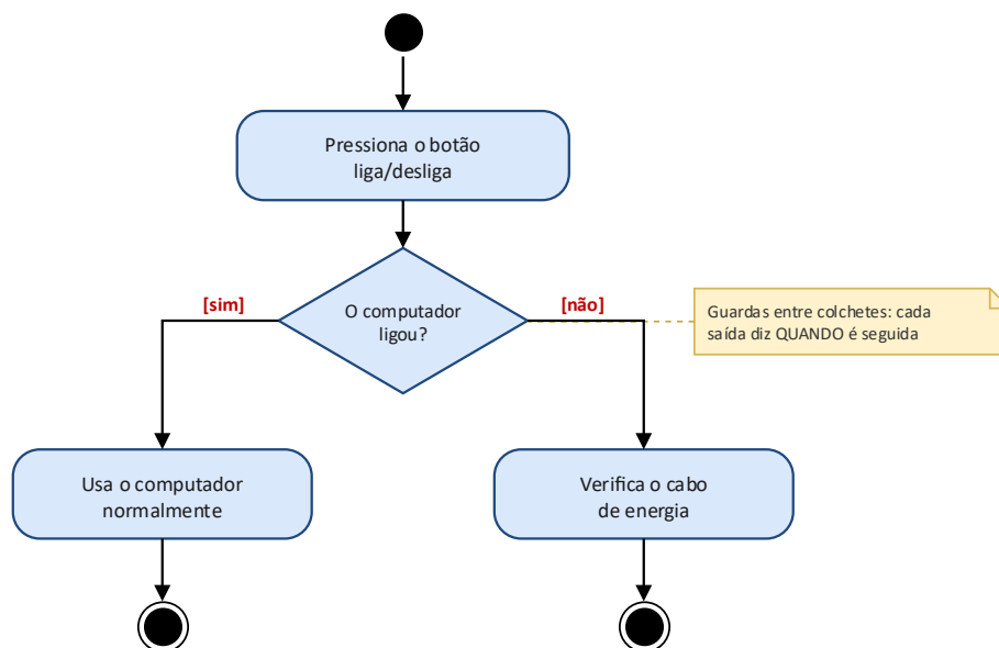
Figura 2 — Diagrama de atividades “ligar o computador”.
